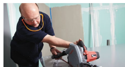
3. Zuschneiden und Bohren
