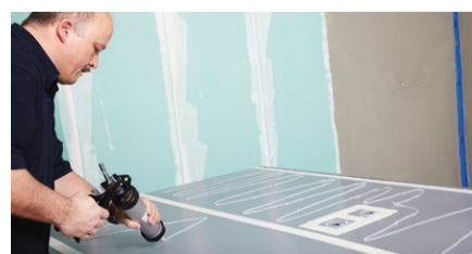
6. Auftragen des Silikons
