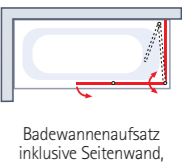
Badewannenaufsatz inkl. Seitenwand, 2-teilig, Anschlag rechts
